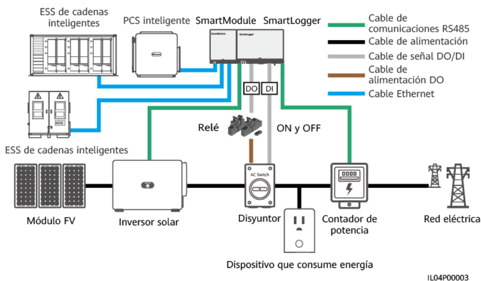
Figura 6-75 Diagrama de red (con un disyuntor)
