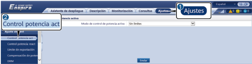
Figura 6-71 Control de potencia activa
