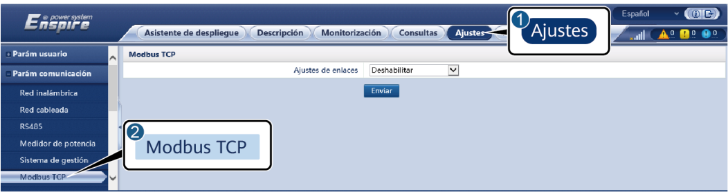
Figura 6-39 Configuración de los parámetros de Modbus TCP
